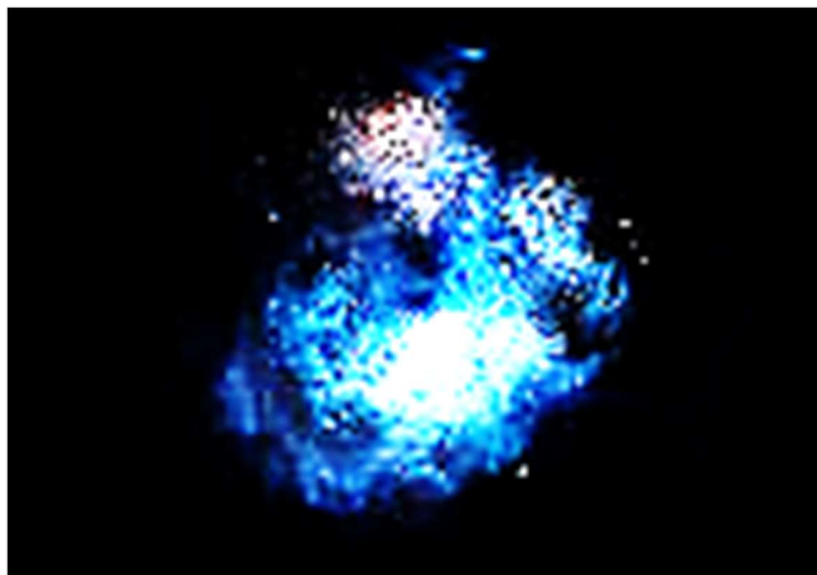
Cosmos Redshift 7 - Constelația -Sextantul. Numele acestei galaxii se bazează pe o deplasare spre roșu z măsurată de aproape 7 (de fapt, z=6,604 ) Galaxia Cosmos Redshift 7 este cea mai strălucitoare dintre galaxiile îndepărtate ( z > 6 ) și conține unele dintre cele mai vechi stele (prima generație; Populația III) care au produs elementele chimice necesare pentru formarea ulterioară a planetelor și a vieții.
